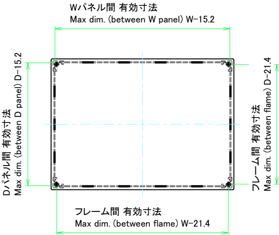
下カバー / Bottom cover
