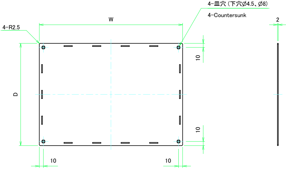
上カバー表面 / Top cover Frontside
