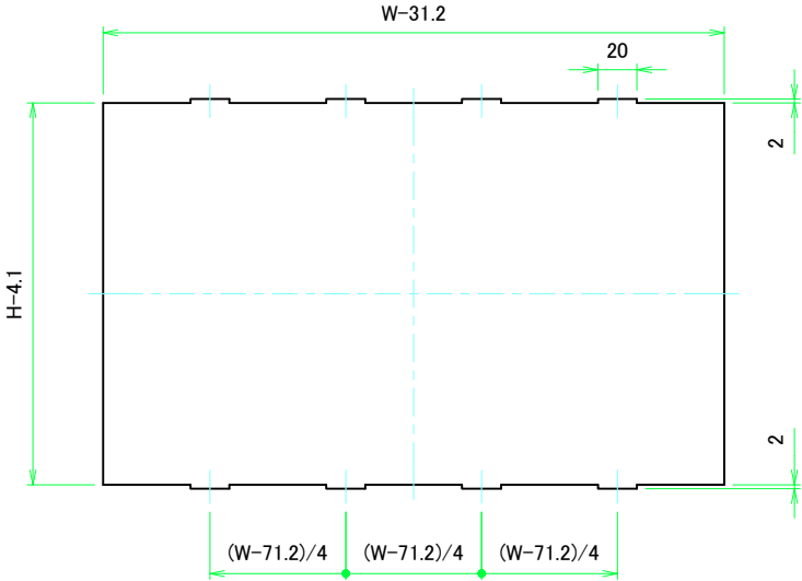
Wパネル1表面 / W Panel 1 Frontside
